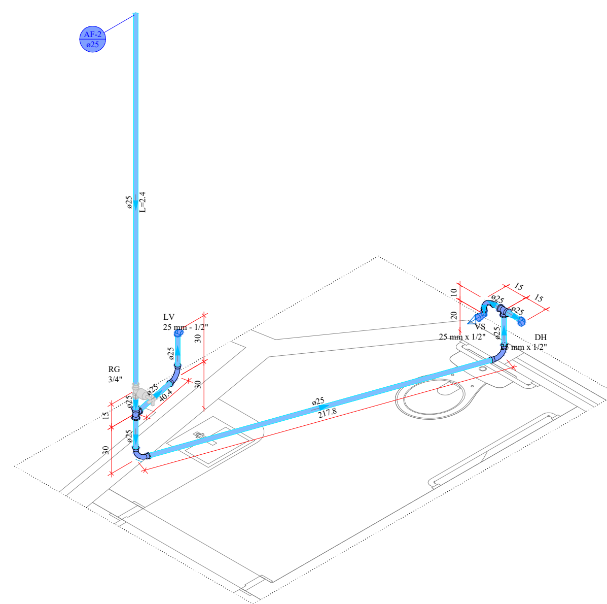
DETALHE Isométrico 2 1:25
