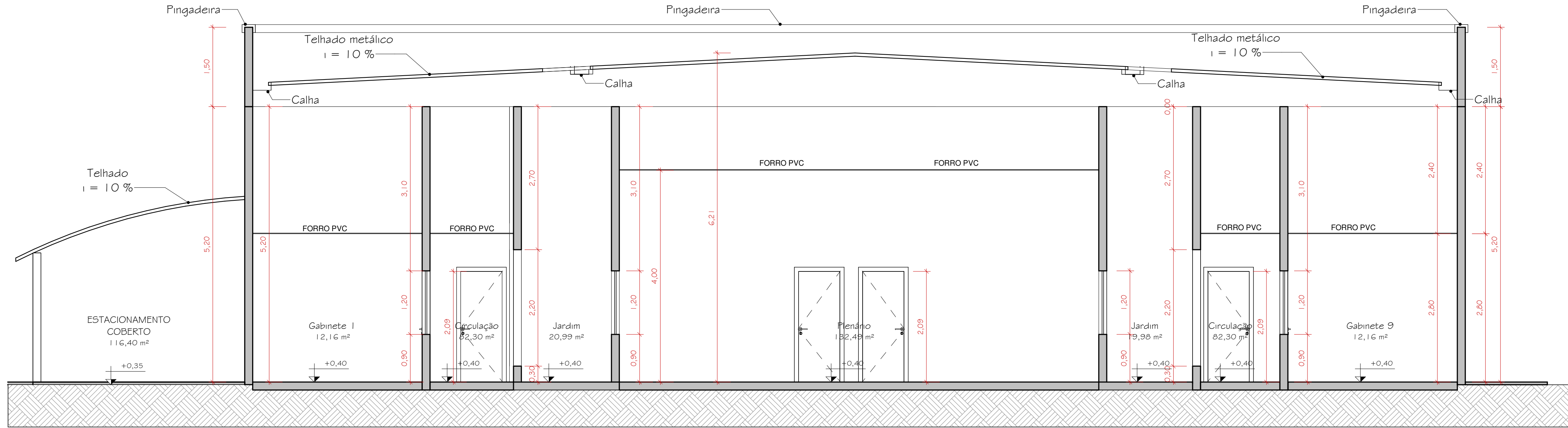
3 Corte B ESCALA: 1:50
