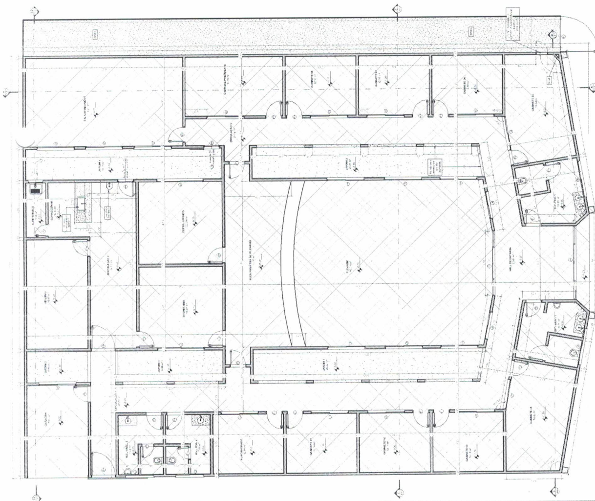
1 PLANTA BAIXA - FINAL 1:50
